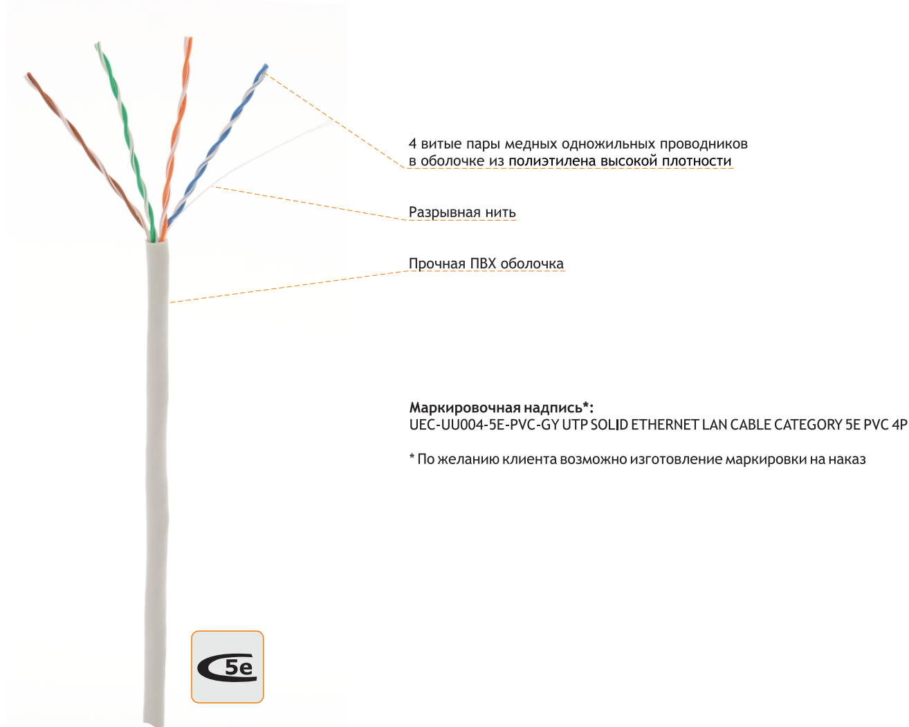
UEC-UU004-5E-PVC-GY
