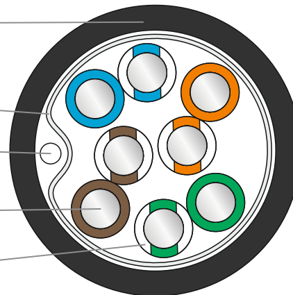
U/UTP
