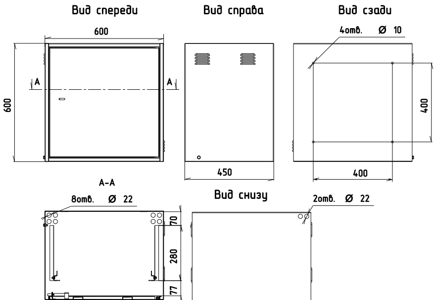
Чертеж шкафа
