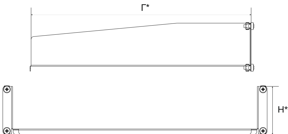
Технический эскиз
